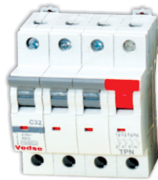
TPN MCB
